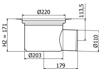
Sida Ø110 mm (Syrast rostfritt stål)
