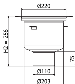
Botten Ø110 mm (Syrast rostfritt stål)
