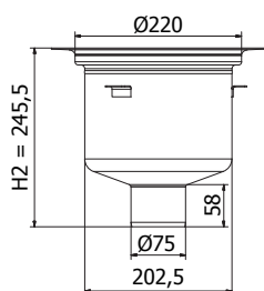
Botten Ø75 mm (Syrast rostfritt stål)
