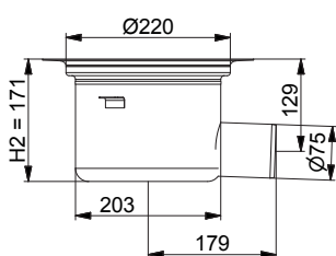
Sida Ø75 mm (Syrast rostfritt stål)
