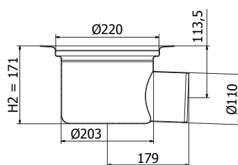
Sida Ø110 mm (Syrafast rostfritt stål)
