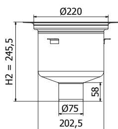
Botten Ø75 mm (Syrafast rostfritt stål)
