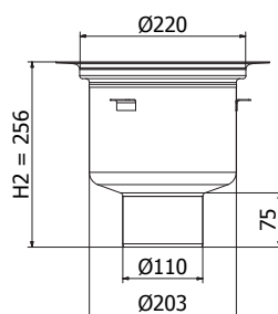
Botten Ø110 mm (Syrafast rostfritt stål)
