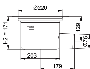
Sida Ø75 mm (Syrafast rostfritt stål)
