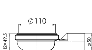
Sida Ø50 mm (PP)
