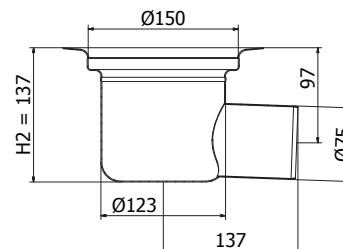
Sida Ø110 mm (Syrafast rostfritt stål)
