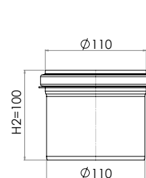
Botten Ø110 mm (Syrafast rostfritt stål)
