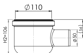
Sida Ø50 mm (PP)
