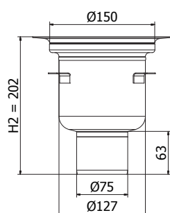
Botten Ø75 mm (Syrafast rostfritt stål)
