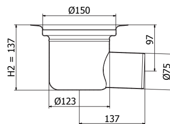
Sida Ø75 mm (Syrafast rostfritt stål)
