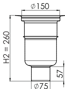
Botten djup Ø75 mm
