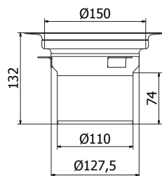
Botten Ø110 mm (Syrafast rostfritt stål)
