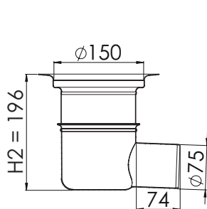
Sida djup Ø75 mm
