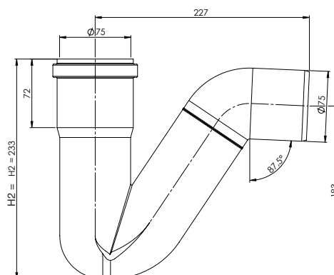
P-vattenlås \varnothing 75 mm (PP)
