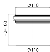
Botten \varnothing 110 mm (Syrast rostfritt stål)
