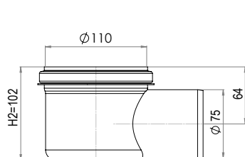
Sida \varnothing 75 mm (Syrast rostfritt stål)
