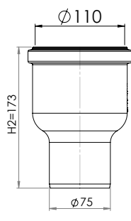
Botten \varnothing 75 mm (PP)
