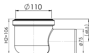
Sida \varnothing 75 mm (PP)
