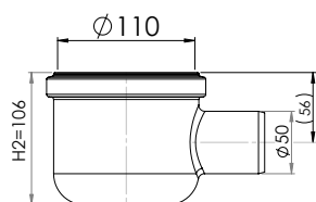
Sida \varnothing 50 mm (PP)
