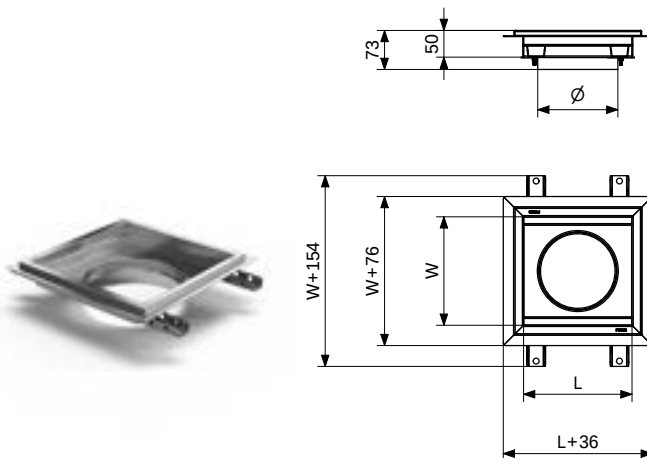
Overdel til epoxygulv
