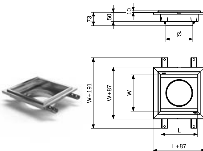
Overdel til klinkegulv
