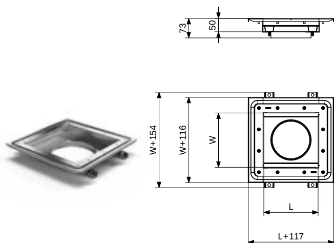
Overdel til vinylgulv
