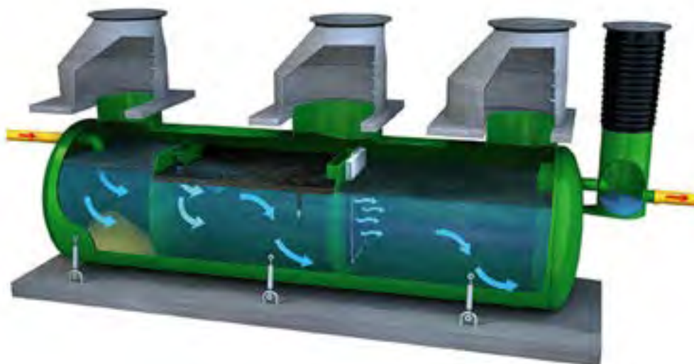
Eksempel på en Klasse I olieudskiller med slamfang og coalescenselement, testet og godkendt efter EN 858-1 og CE mærket.
