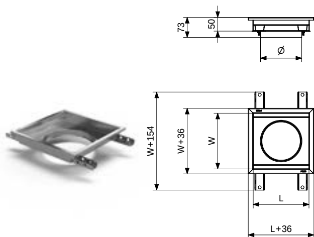
Overdel til betongulv
